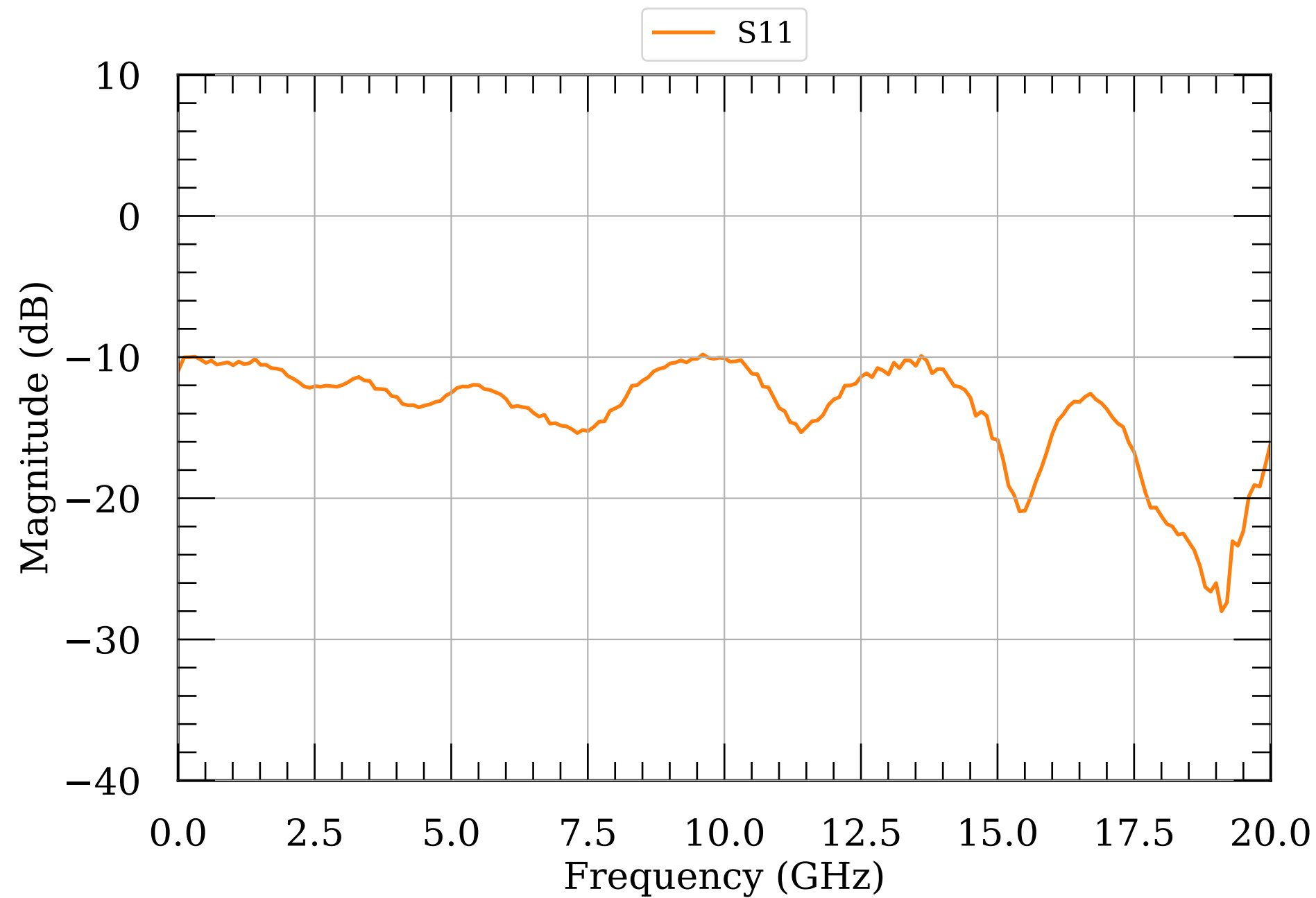
LNA S-params module056
